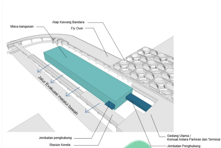
Gambar.2.7 Masa bangunan terhadap tapak. Sumber : Analisis Penulis, 2021
