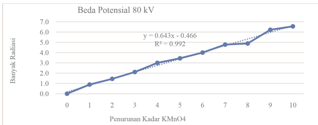
Gambar 3. Grafik Peningkatan Radikal Bebas pada Air dengan Bada Potensial Sebesar 80 kV
