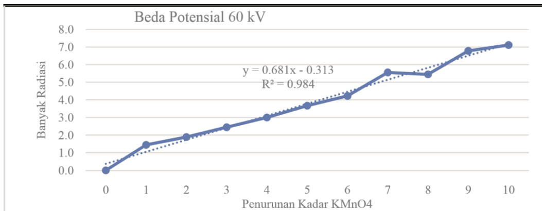
Gambar 2. Grafik Peningkatan Radikal Bebas pada Air dengan Bada Potensial Sebesar 60 kV
